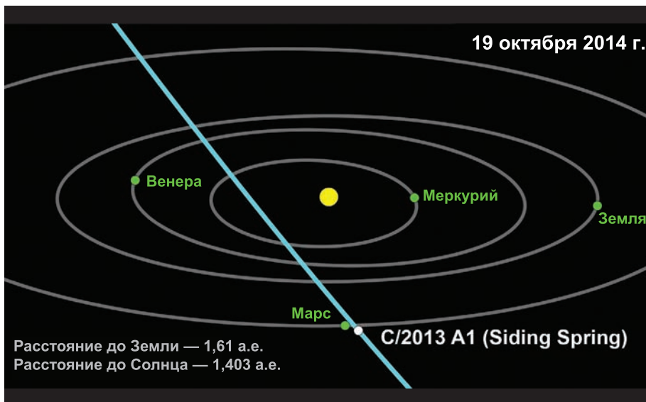
Схема, показывающая ориентацию орбиты кометы C/2013A1 Siding Spring относительно орбит внутренних планет Солнечной системы и их положение по состоянию на середину октября 2014 г.
