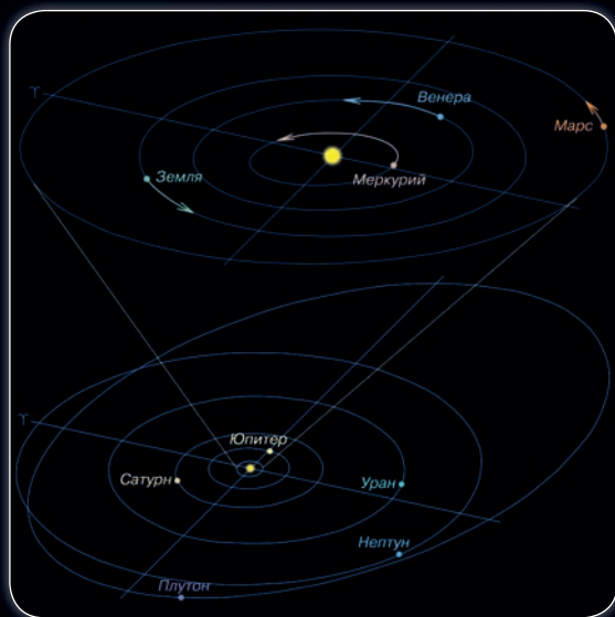
Положения планет на орбитах в мае 2013 г.
