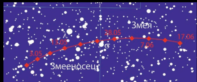
Видимый путь астероида Геба (6 Hebe) в мае-июне 2013 г.
